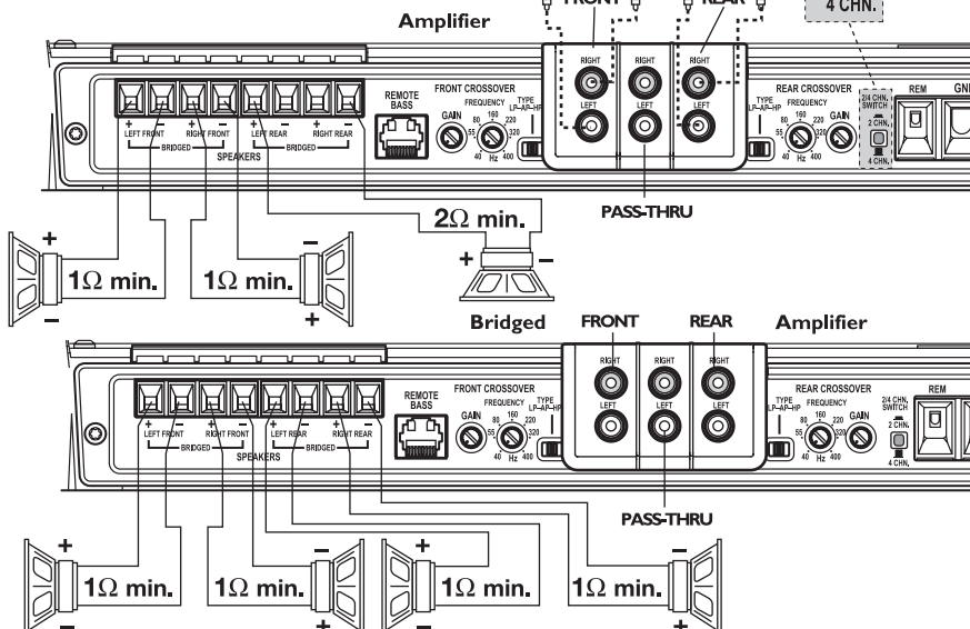
Câblage à 4 voies
