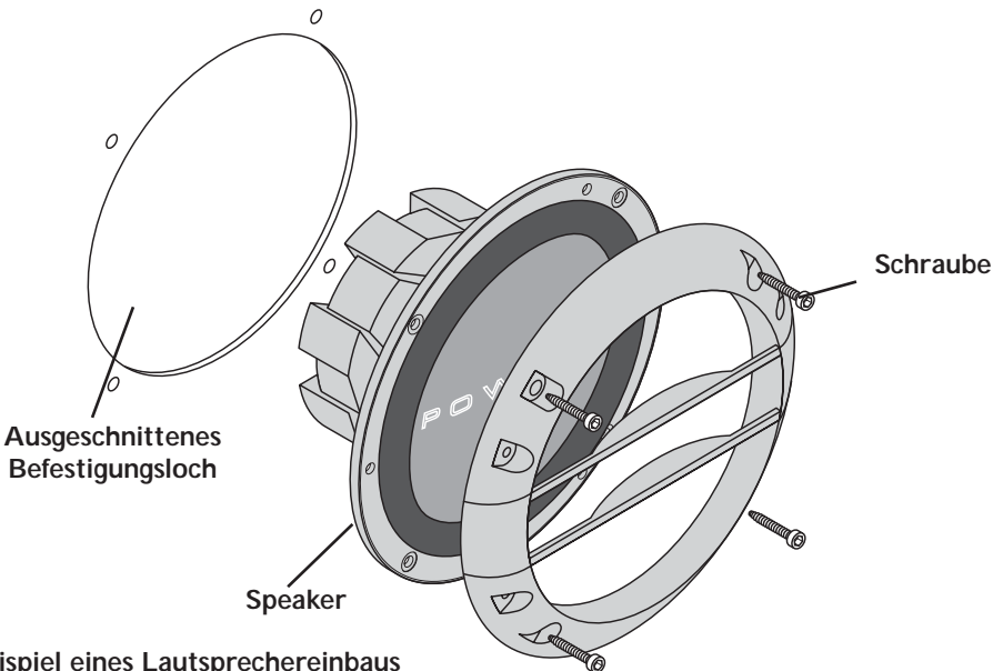
Beispiel eines Lautsprechereinbaus
