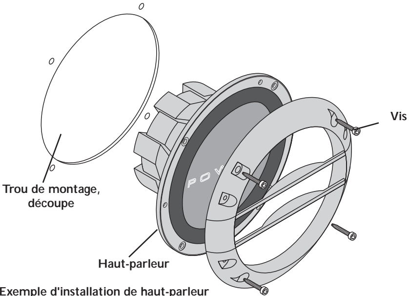
Exemple d'installation de haut-parleur
